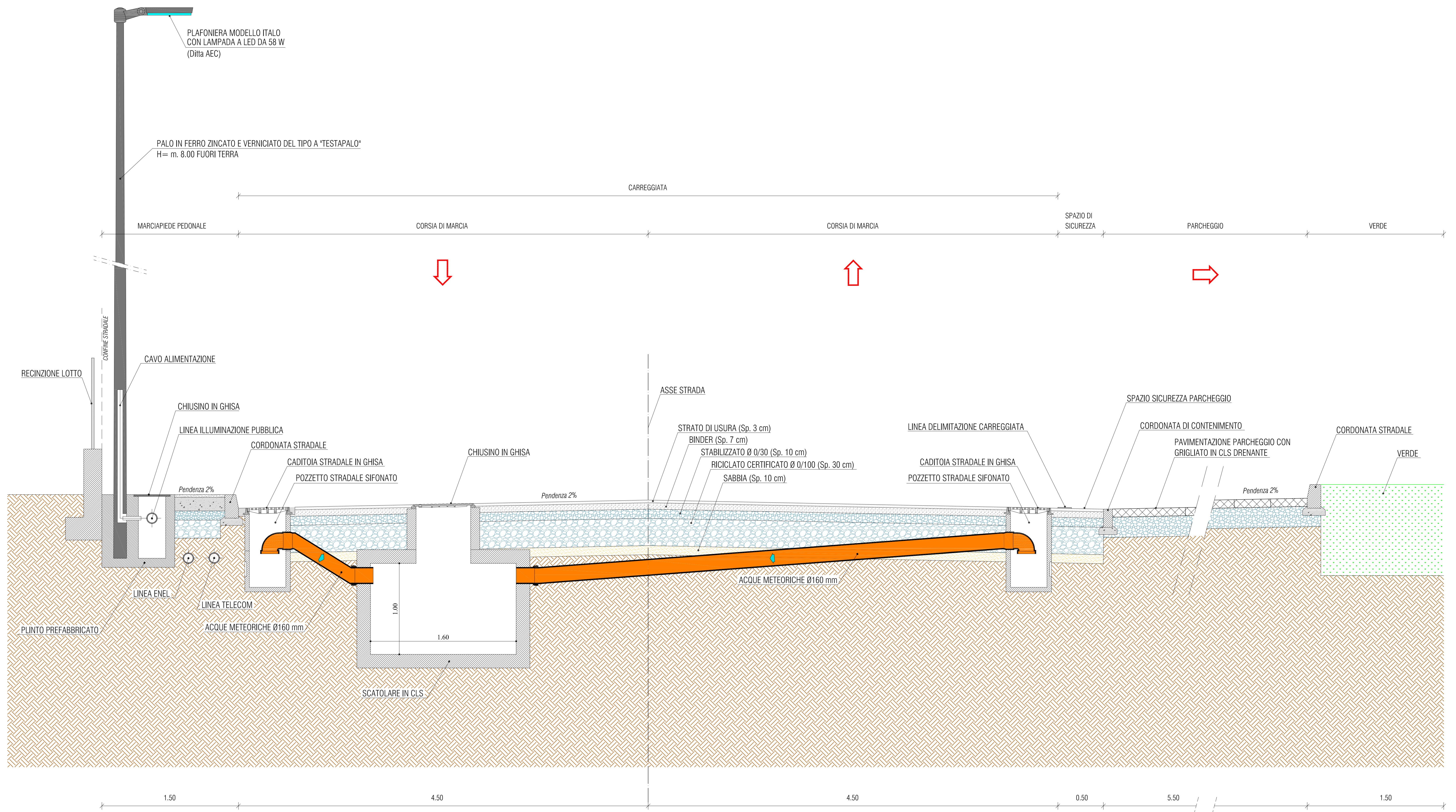
SEZIONE STRADALE TIPO Scala 1:20
